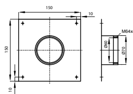
1. Króciec Pomiarowy
