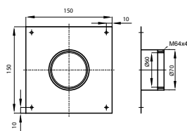
1. Króciec Pomiarowy
